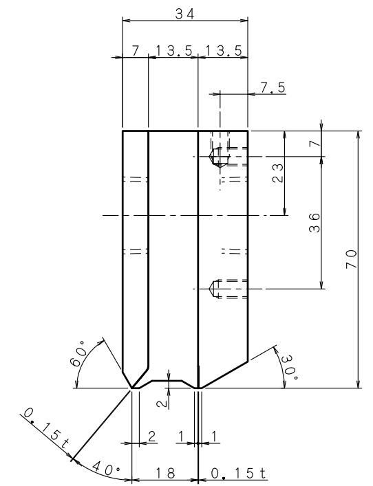
A矢視拡大図
